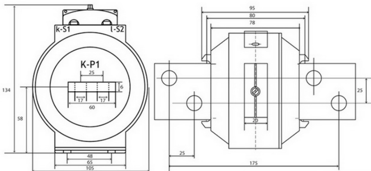
AMT-0-V 750/5-1000/5
