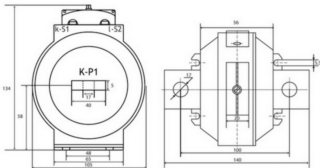
AMT-0-V 400/5-600/5
